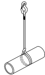
Figure D.2 — Élingage baguë double
