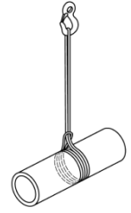
Figura C.1 — Attacco a doppia fascia
