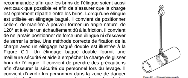
Figure C.1 — Élingage bagué double
