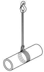
Figure C.1 — Élévation à deux bandes
