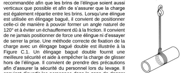
Figure C.1 — Élingage bagué double
