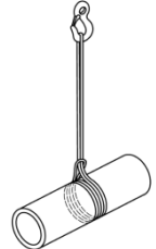
Figure C.1 — Elévation à deux bandes
