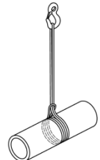
Figure C.1 – Elingage boguée double
