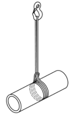
Figure C.1 – Élévation à deux pennes
