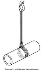
Figure C.1 — Élingage bagué double
