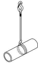
Figure D.2 — Élingage baquet double
