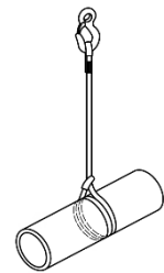
Figure D.2 — Élingage bague double
