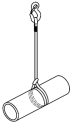
Figure D.2 — Élingage boucle double
