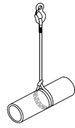
Figure D.2 — Élingage bagué double
