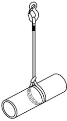
Figure D.2 — Élingage baigué double
