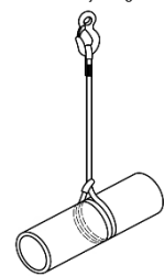
Figure D.2 — Élingue baguet double
