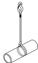
Figure D.2 — Élingage baguette double
