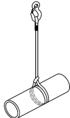
Figure D.2 — Élingage baigué double
