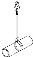
Figure D.2 — Élingage bague double
