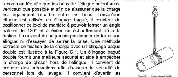
Figure C.1 — Élingage bagué double
