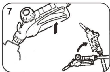
7 Remova o bico do recipiente
